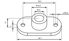
Upper Hinge and Striker Üst menteşe karşılığı
